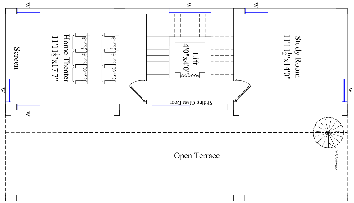
S.F. Plan Slab Area : 744.533 Sq.Ft.
